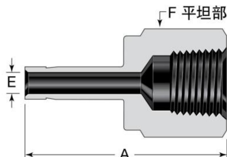
英制Tube管 Fractional Tube
