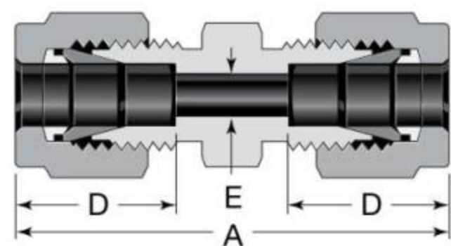
英制Tube管 Fractional Tube
