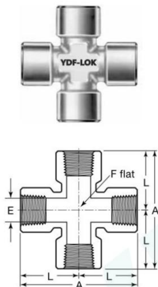
内牙四通 (Crosses)
