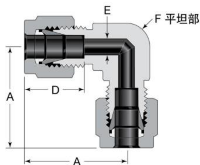
英制Tube管 Fractional Tube
