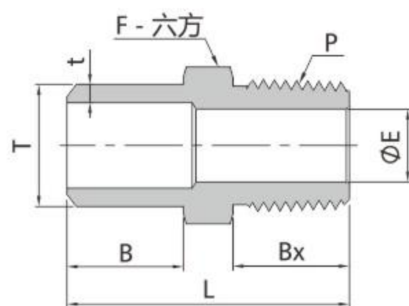
Tube 管对焊-阳螺纹接头
