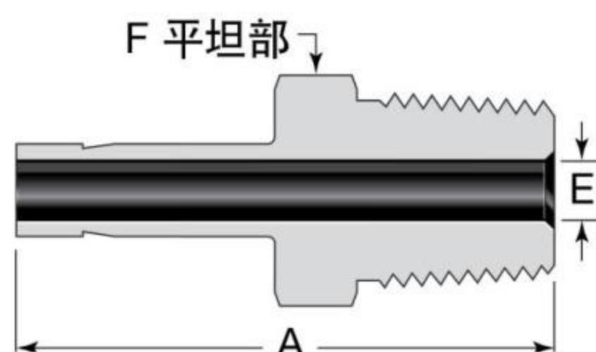
英制Tube管 Fractional Tube
