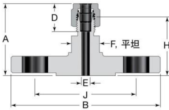
英制Tube管 Fractional Tube
