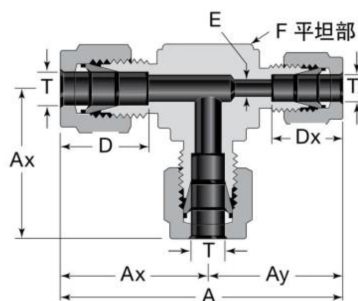
英制Tube管 Fractional Tube
