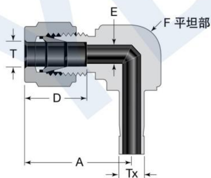
公制Tube管 Metric Tube
